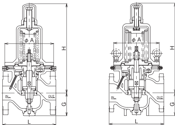
呼び径15～80
