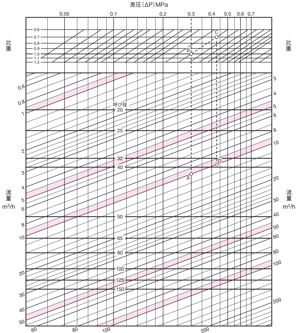
呼び径選定図表(液体用)
