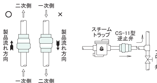
図1. 垂直配管取付姿勢
