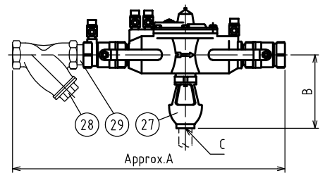
エアギャップおよびストレーナ取付図 INSTALLATION OF AIR GAP AND STRAINER
