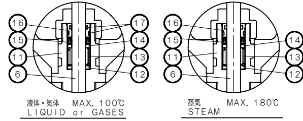
矢視 (A) 部 パッキングランド部構造 CONSTRUCTION OF PACKING GLAND (A PORTION ABOVE)
