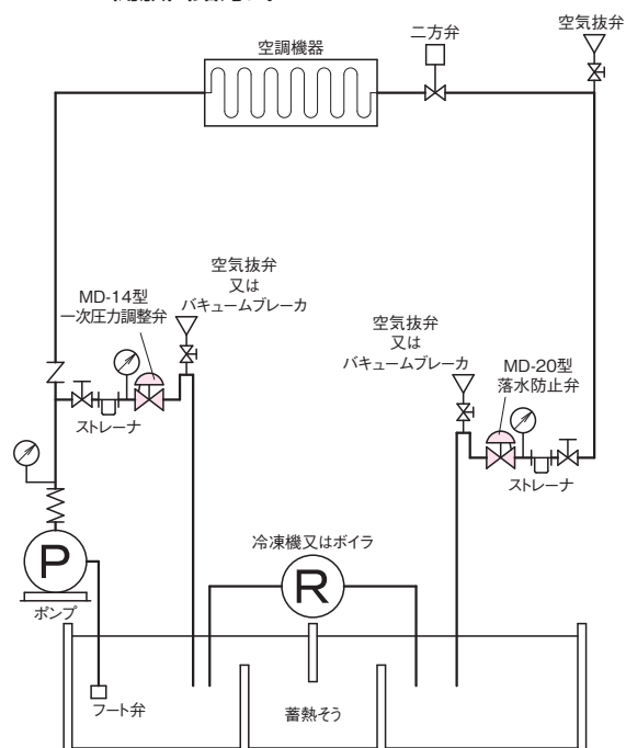
開放回路方式
