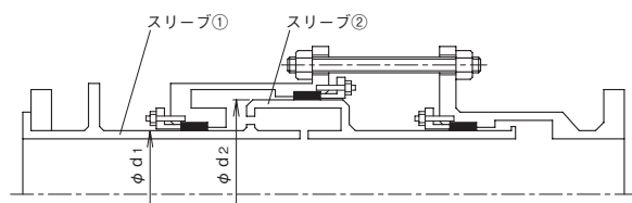
図5. 圧力バランス形
