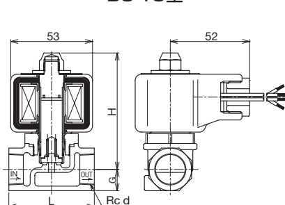
DS-15型
