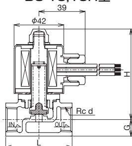
DS-10,10H型
