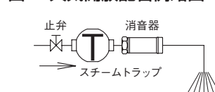
図8. 機器取付例略図
