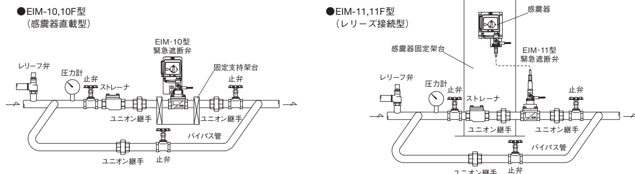
図1. 配管例略図
