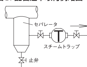
図4. 管末取付例略図
