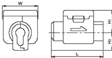
寸法表
