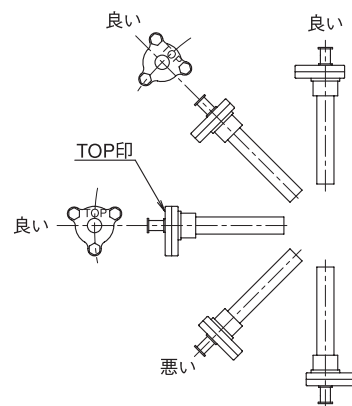
図3. 感熱筒取付け方向
