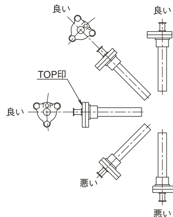
図3. 感熱筒取付け方向
