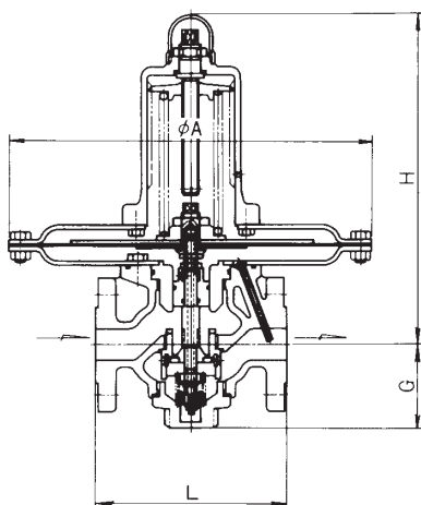
RD-29A型 オリングシール・圧力バランス構造
