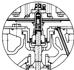
ベロフラムシール・圧力バランス構造
