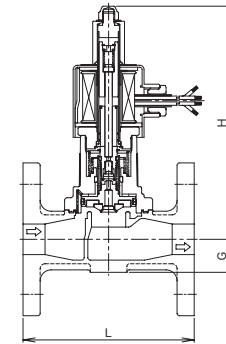
PF-12C型
