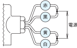
AC100/110Vの場合
