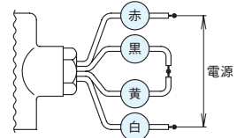
AC200/220Vの場合
