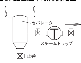
■図4. 管末取付例略図
